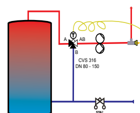
Montage DN 80 - 150
