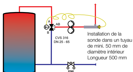
Montage DN 25 - 65
